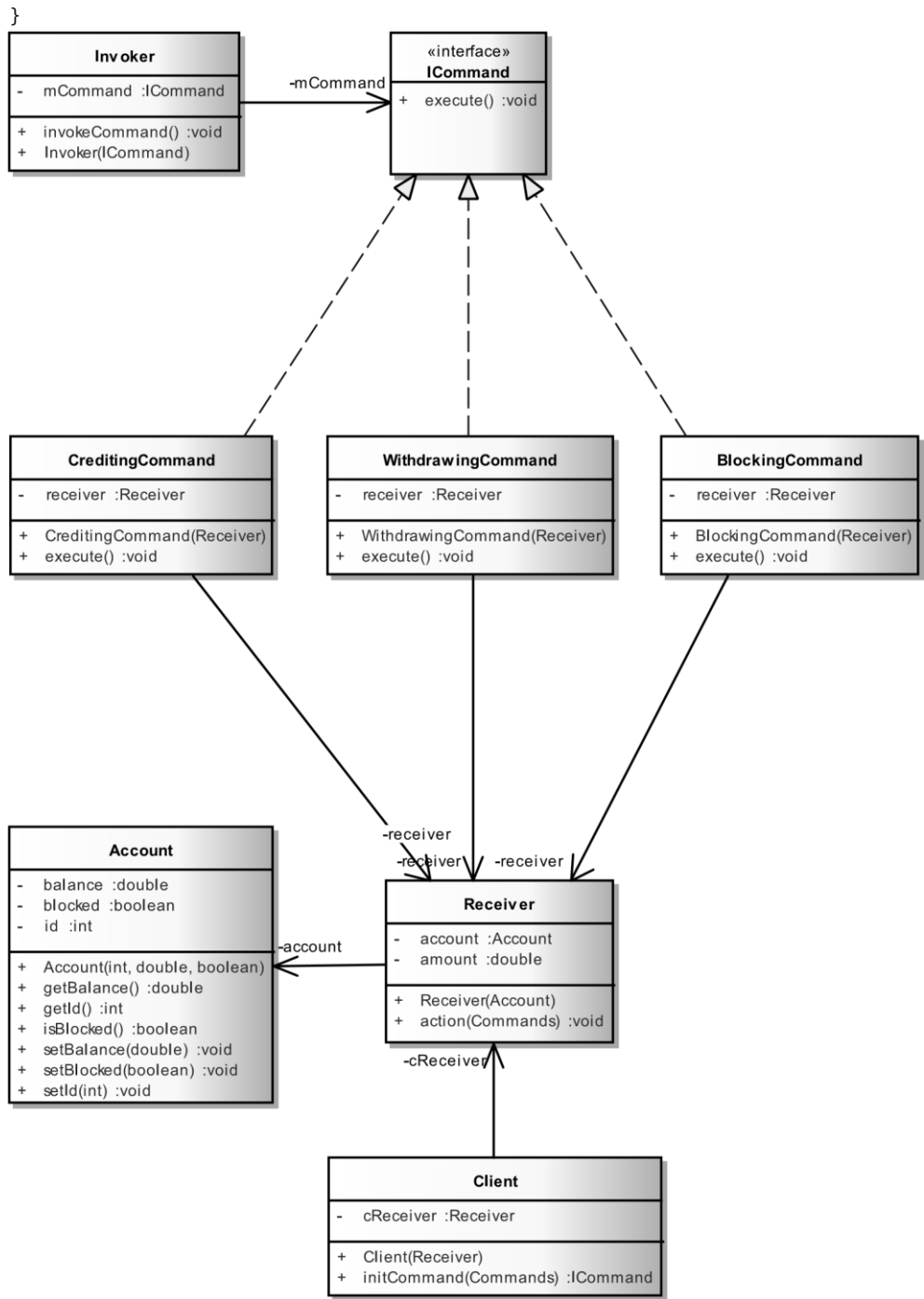
Рис. 22.5. Реализация шаблона Command
