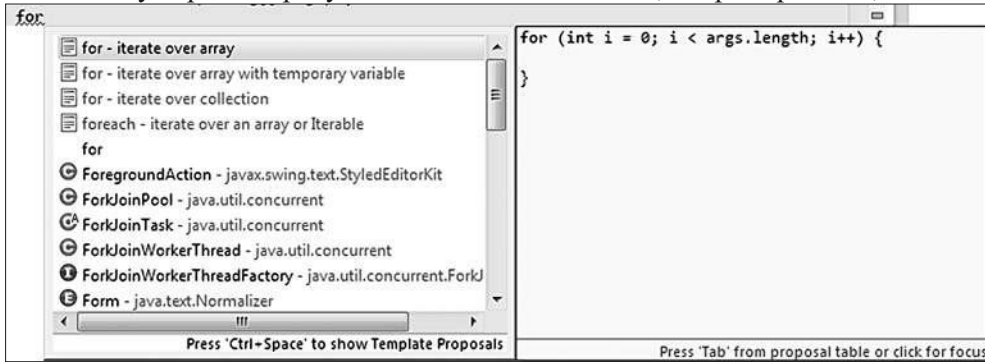
Рис. 24. Вызов шаблона
