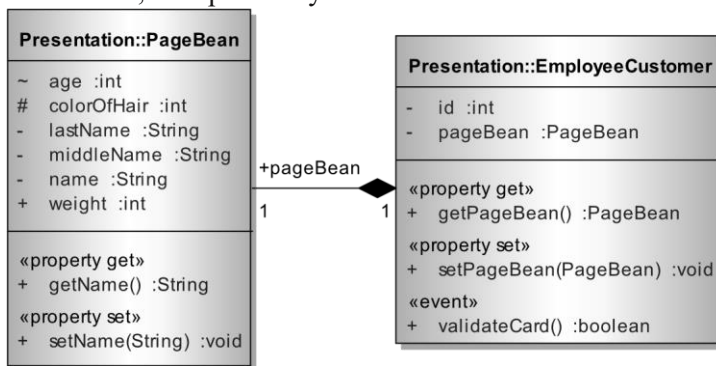
Рис. 9. Множественность
