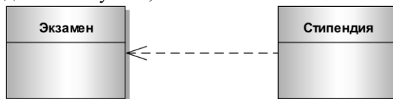
Рис. 4. Отношение зависимости
