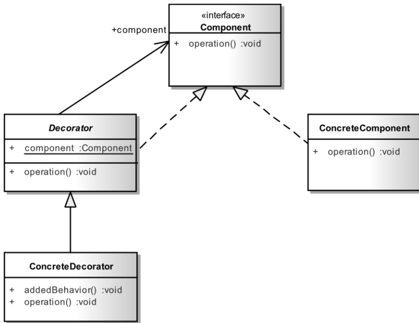
Рис. 23.3. Базовая реализация шаблона Decorator
