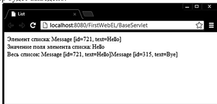
Рис. 16.3. Использование EL для доступа к элементам списка
