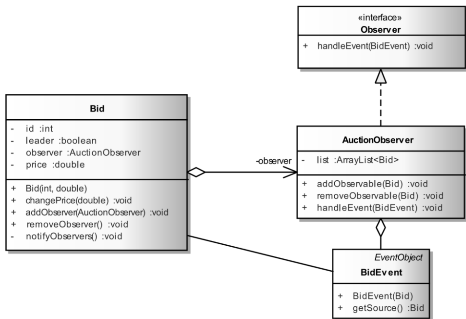
Рис. 22.12. Пример реализации шаблона Observer
