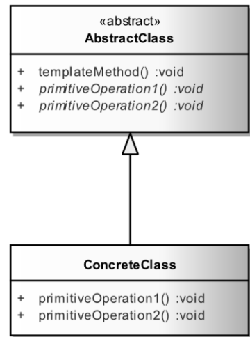
Рис. 22.17. Базовая реализация шаблона Template Method
