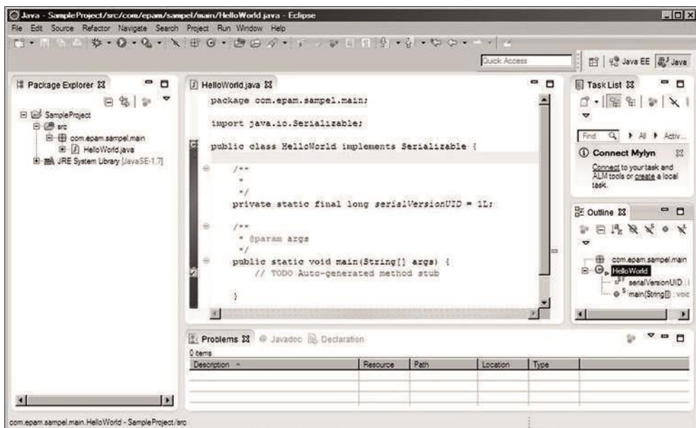
Рис. 9. Сгенерированный класс
