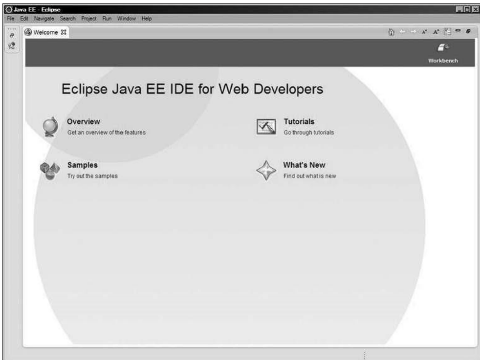
Рис. 2. Welcome page
