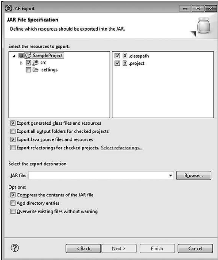
Рис. 31. Экспорт проекта
