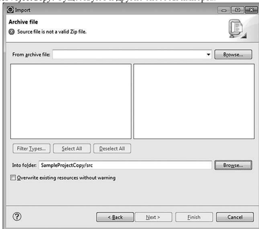
Рис. 32. Импорт проекта
