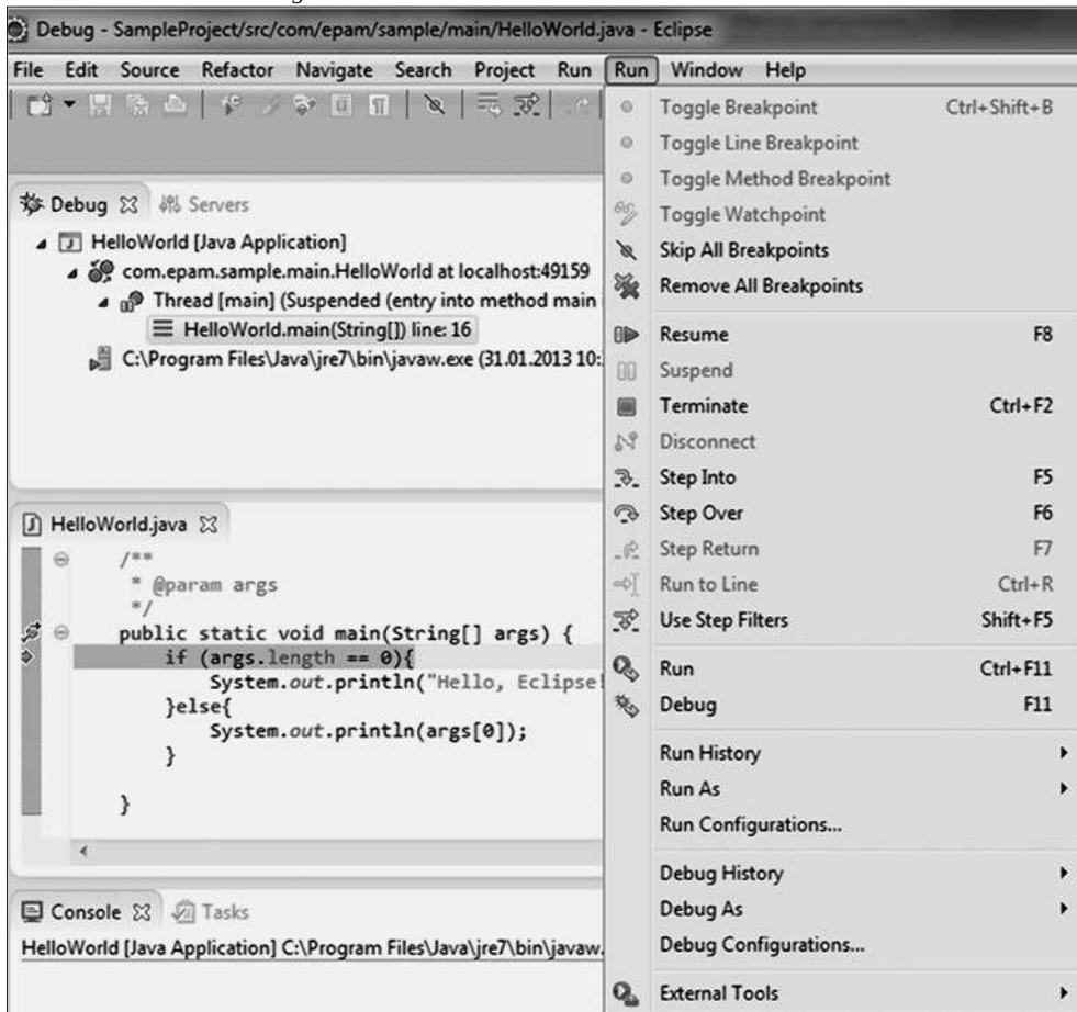
Рис. 13. Управление отладкой
