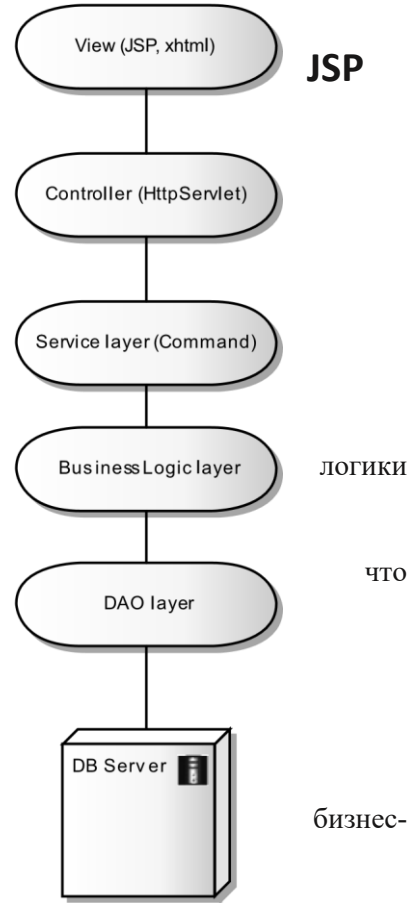
Рис. 16.7. Вариант
